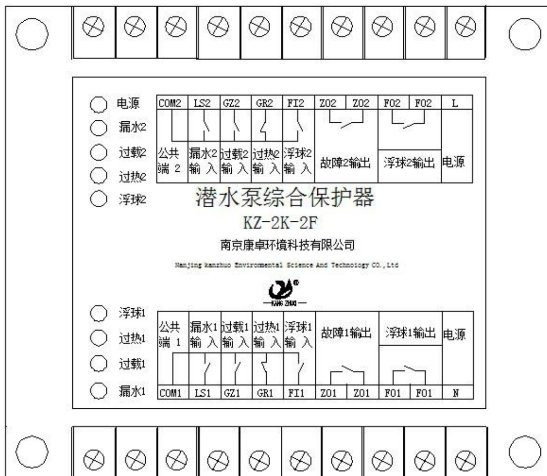
(2) 面板示意图
